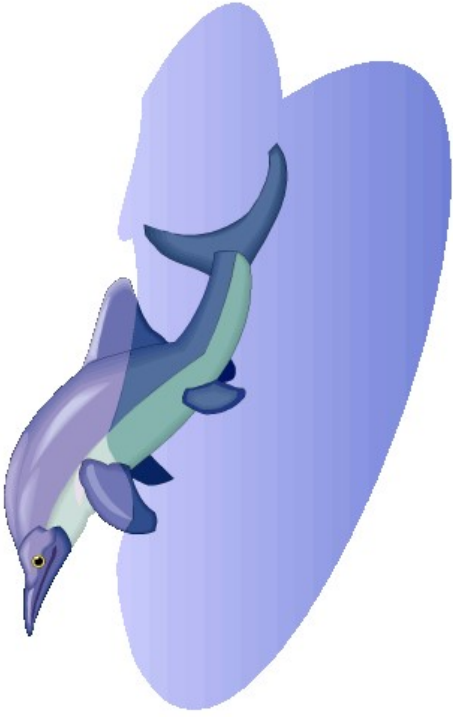
Ichthyosaurus
