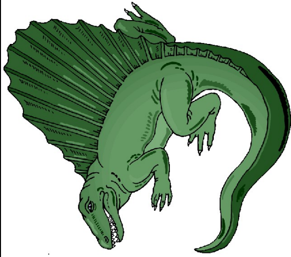
Dimetrodon
